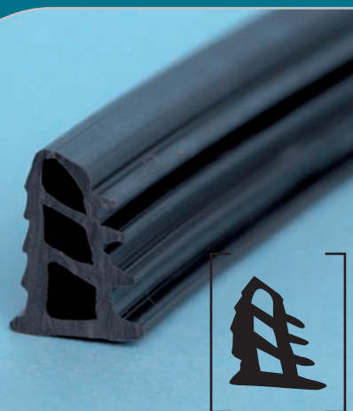
GOMA MODELO HUECA
